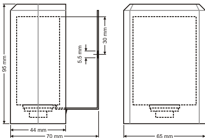
Fig. 1. Dimensions (mm)
